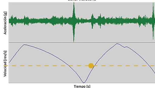
Señal vibratoria
